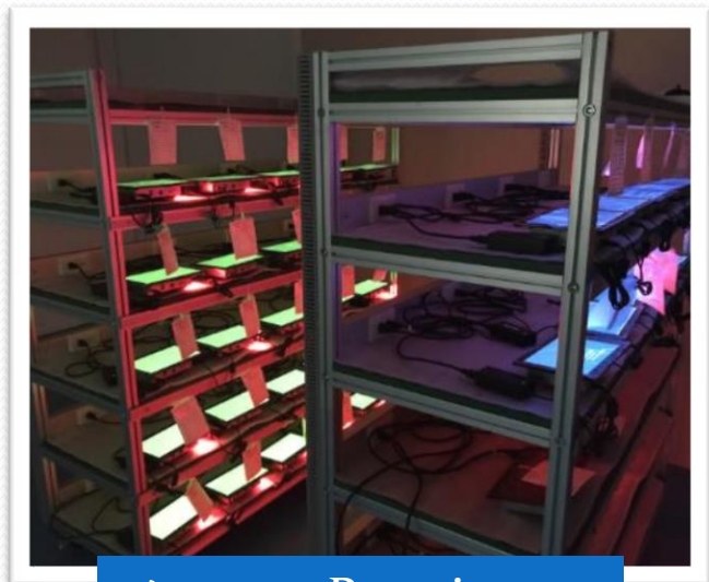
系統測試/Burn in test
