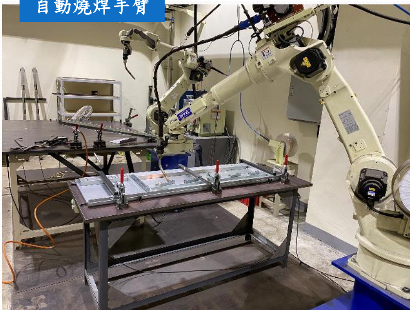
自動燒焊手臂
